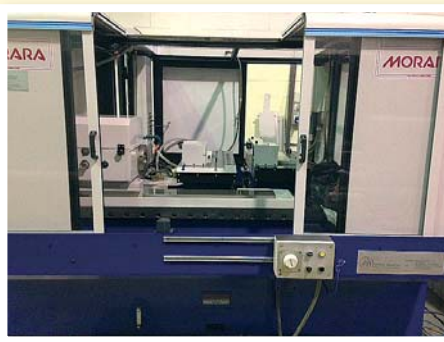
▲ Centro di rettificazione MORARA INTERMATIC 1000 CNC 750 R NUM a due carri I + I oppure I + E
